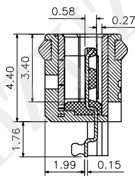
SECTION:A-A SCALE 1:1
